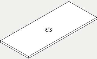
170×70×H2 cm SDPD17007020 170×80×H2 cm SDPD17008020 Piatto doccia 170 cm SoloDue®. SoloDue® shower tray 170 cm.
