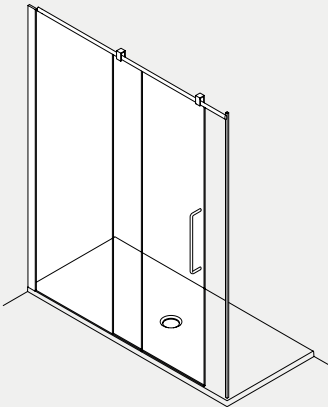
su misura, bespoke CX01 Box doccia in acciaio, 1 anta fissa + 1 anta scorrevole. Steel shower box, 1 fixed door + 1 sliding door.
