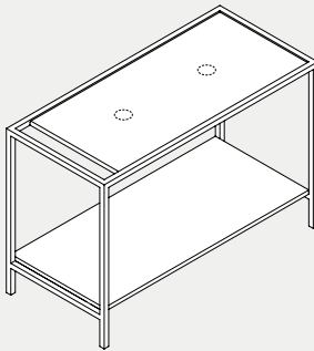
120×55×H80 cm STP 120 04
