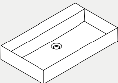
80×45×H12,5 cm ELLP080450Q0
